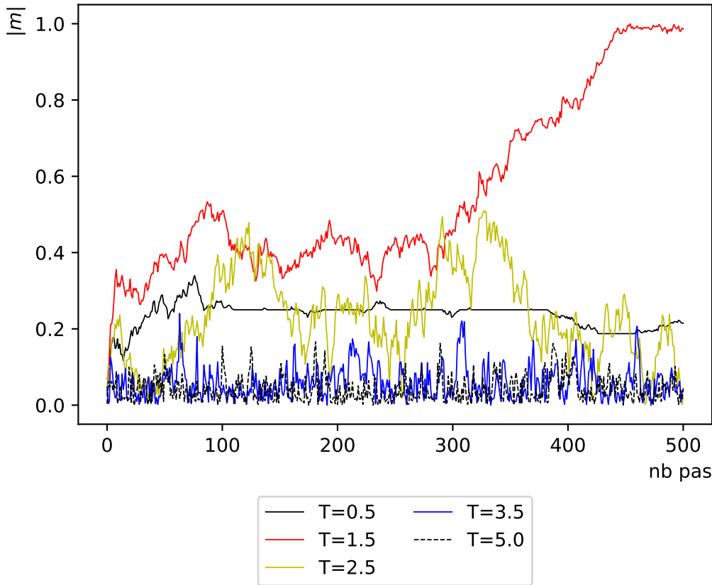
Evolution de l'aimantation sur 500 pas de Monte Carlo, N=32
